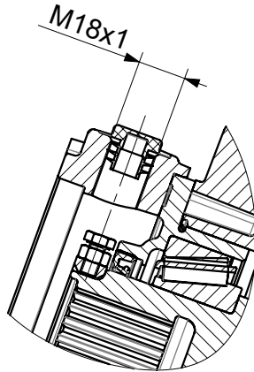
SEZ. B-B
