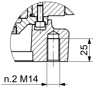
SEZ. A-A
